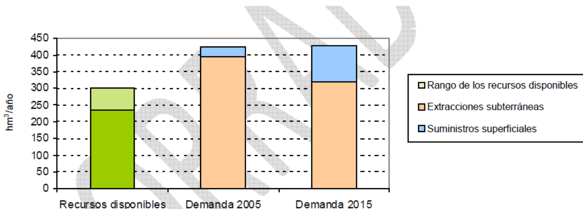
Figura 7. Recursos disponibles, demanda total y extracciones en la masa de agua Mancha Oriental antes y después de la puesta en marcha de las medidas propuestas
